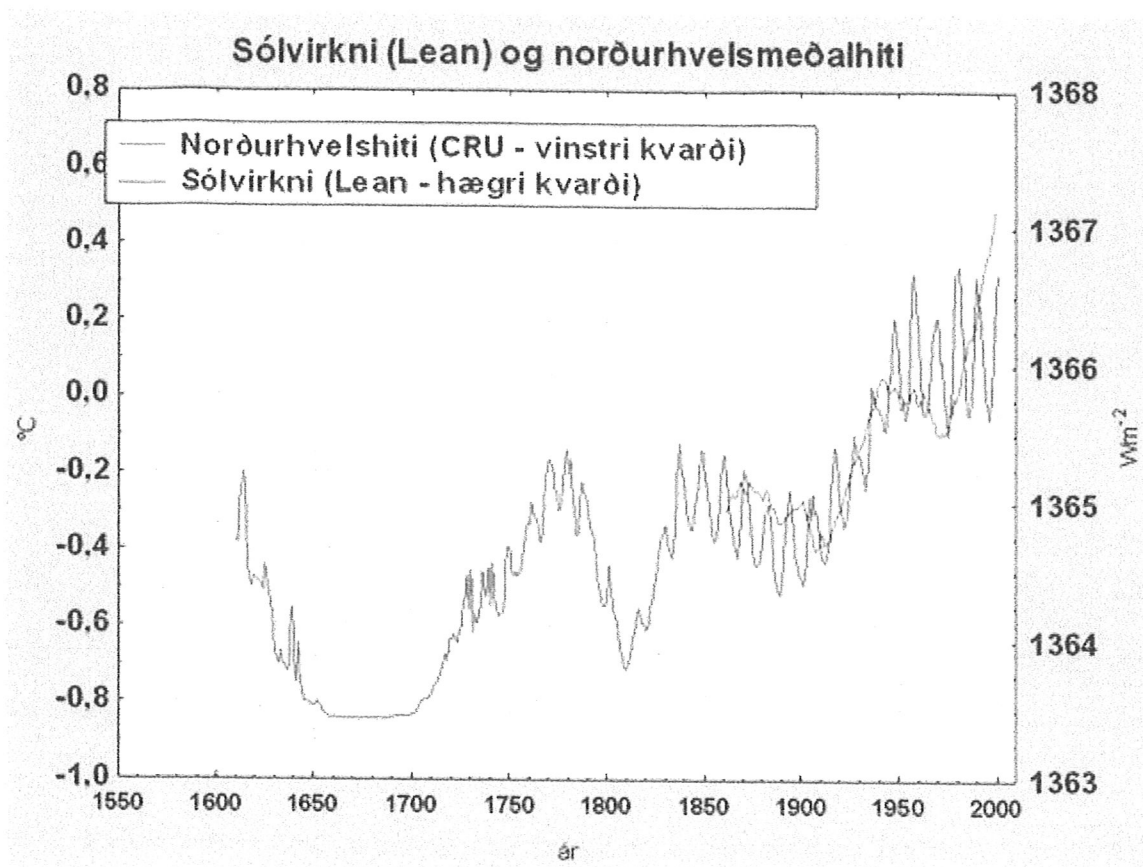
Mynd 6. Virkni sólar 1600 til 2000 (ágiskun Lean ? rauður ferill) ásamt 11-ára keðjumeðaltölum norðurhvelshita (CRU) frá 1856 (blár ferill). Sýnd eru mestu sólblettalágmörkin, hið fyrra á 17. öld, en þá var sólin nánast blettalaus í marga áratugi, en hið síðara snemma á 19. öld. Gögn frá Lean: Lean, J. 2004. Solar Irradiance Reconstruction. IGBP PAGES/World Data Center for Paleoclimatology. Data Contribution Series # 2004-035.
