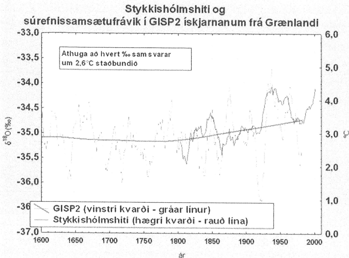
Mynd 5. Samsætufrávik í GISP2-kjarnanum á Grænlandi frá því um 1600. Þunn grá lína sýnir 11-ára keðjumeðaltöl, en sú þykka er útjöfnun (sömu gögn og línur og á mynd 4). Rauða línan sýnir 11-ára keðjumeðaltöl hita í Stykkishólmi frá 1798. GISP2-gögn: Sjá texta með mynd 4.
